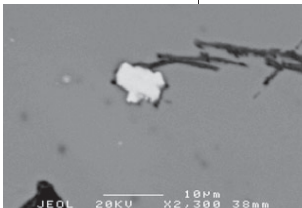
Abb. 28: Hypidiomorphes, winziges Kassiterit-Korn (hell) als Einschluss in Tennantit vom Brunnkendlgraben, Revier Schwarzleo. Sammlung: NHM Wien. REM-Foto (BSE-Modus): F. Brandstätter und U. Kolitsch
