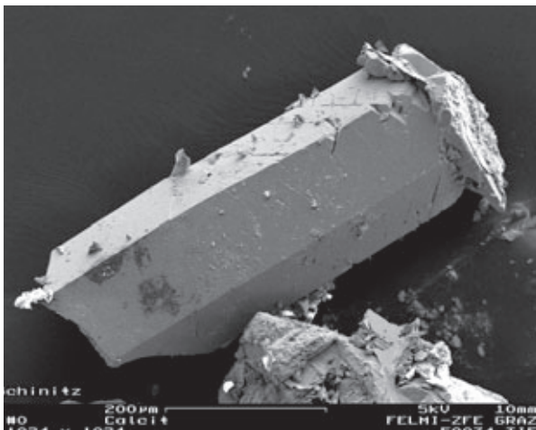
Abb. 36: Calcitkristall mit dominierendem hexagonalem Prisma \{11\bar{2}0\} . Magnesit-Tagbau Kaintaleck. REM-Foto: SE-Modus. Zentrum für Elektronenmikroskopie Graz
