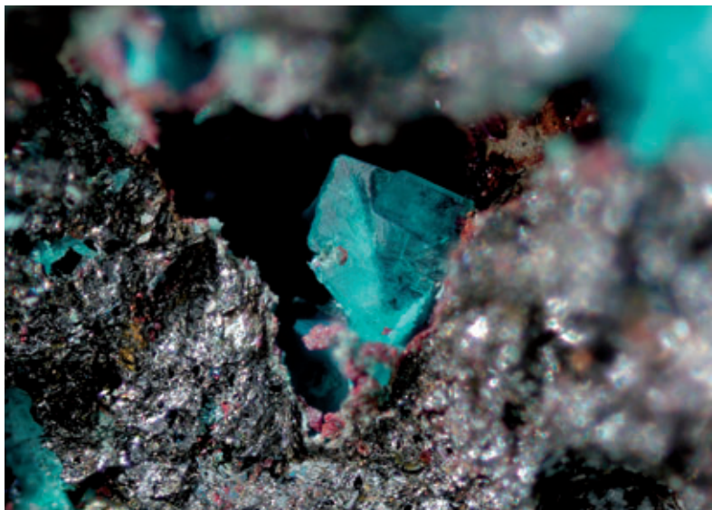
Abb. 1: Hellbläuliche, miteinander ver- wachsene Rouait- Täfelchen (max. 1 mm) auf Schlacken- matrix. Die recht- eckige Begrenzung der Täfelchen ist im Foto nur schlecht erkennbar. Sammlung: P. Hubert. Foto: S. Wolfsried
